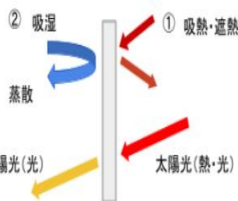
2018年度 蒸散作用を持った遮熱カーテン
